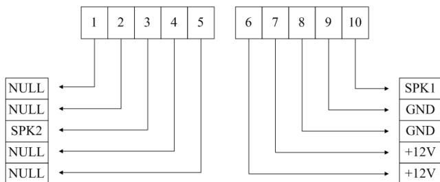
G395 端子图
